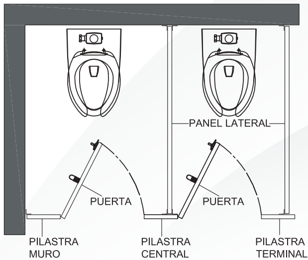
VISTA SUPERIOR
